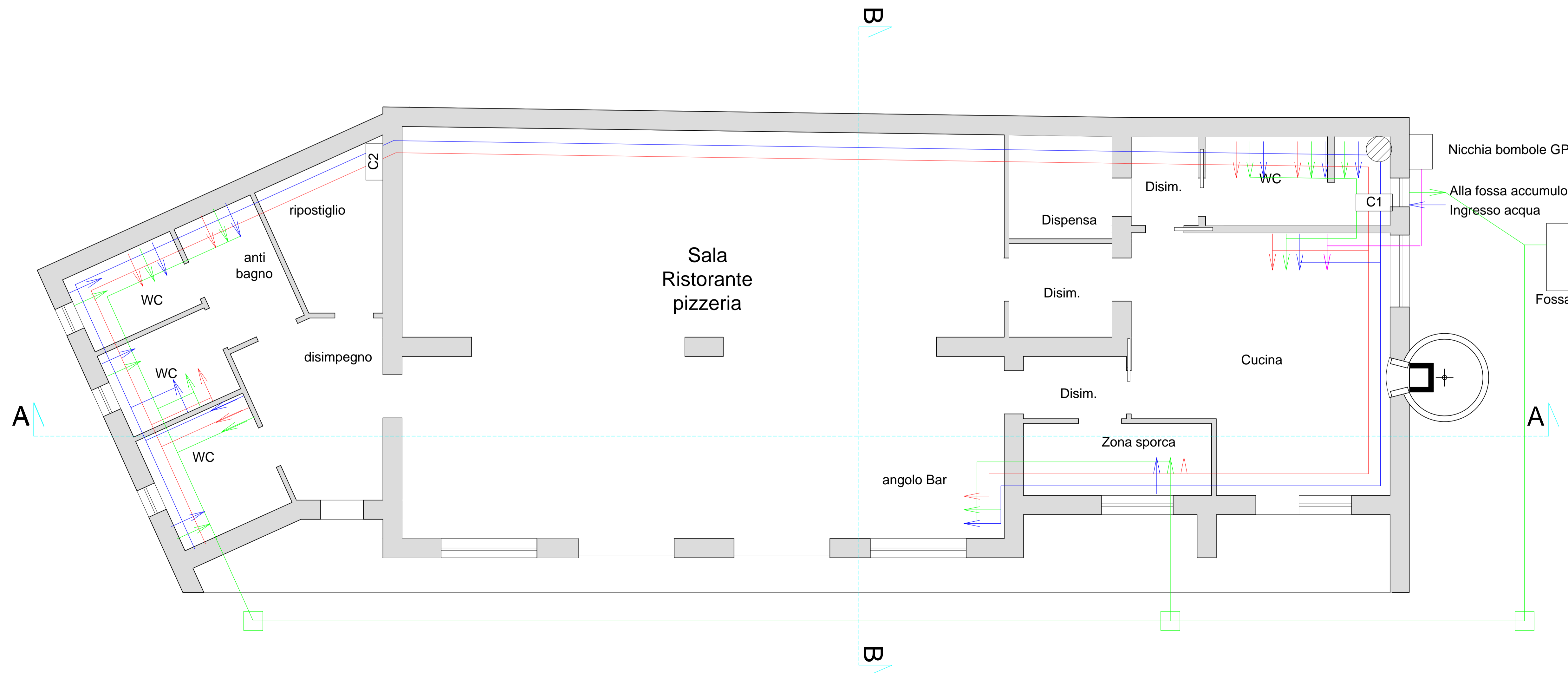
PIANTA IMPIANTO IDRAULICO
