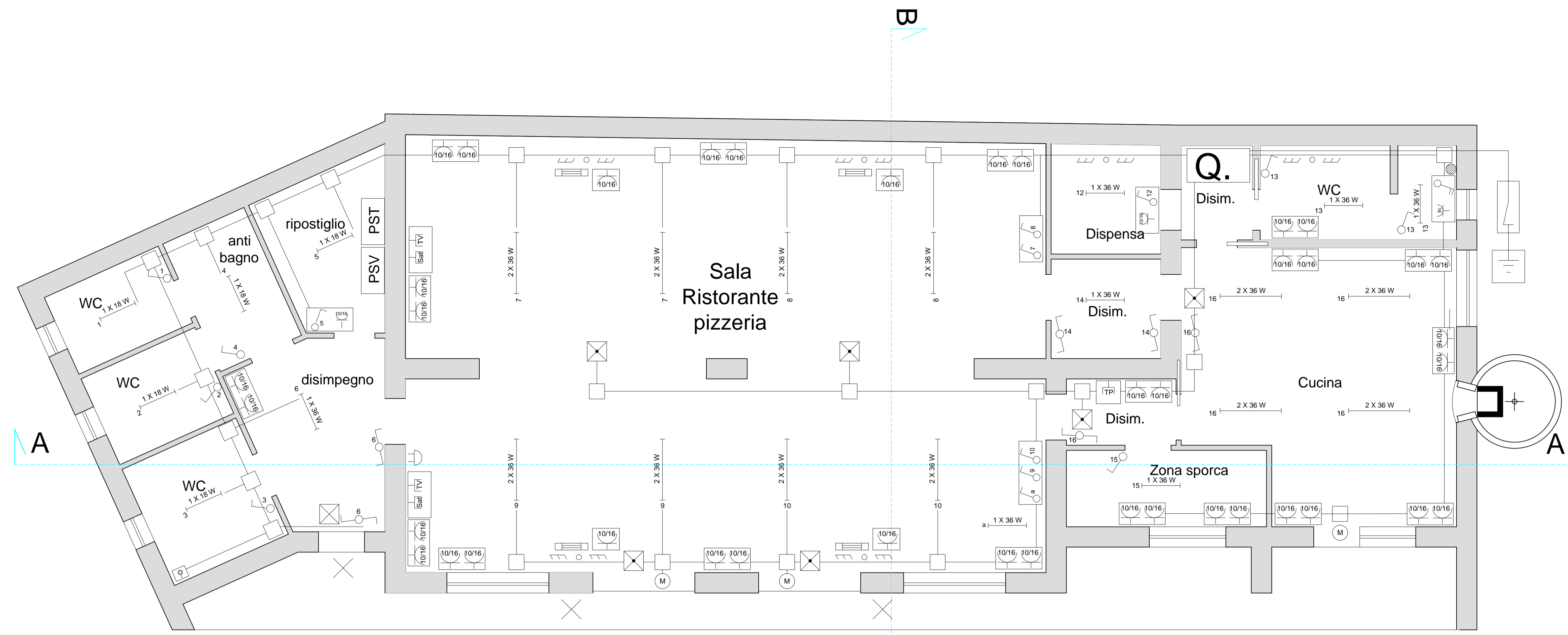
PIANTA IMPIANTO ELETTRICO
